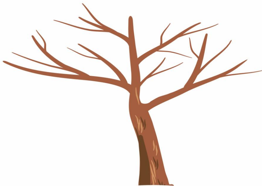
Рисунок 2 «Дерево безопасности»
